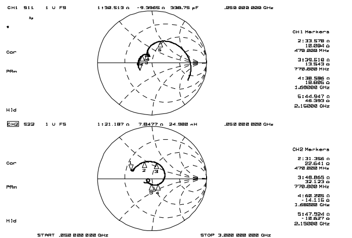
Zin, Zout
