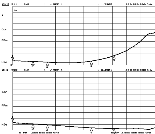
VSWR
