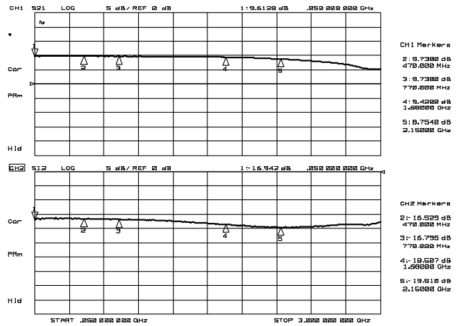
S21, S12
